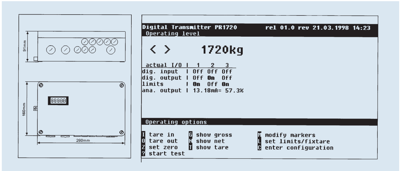
Dimensions PR 1720
